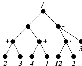
Kuva 5.15. Laskutoimituspuu.
