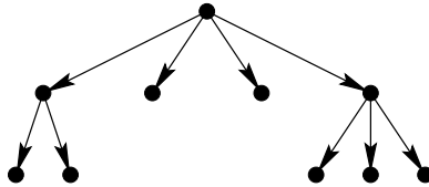
Kuva 5.2. Juurellinen puu.
