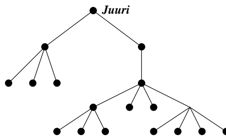
Kuva 5.5. Juurellinen 4-puu.
